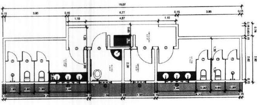
3 PLANTA BAIXA 1 : 50
